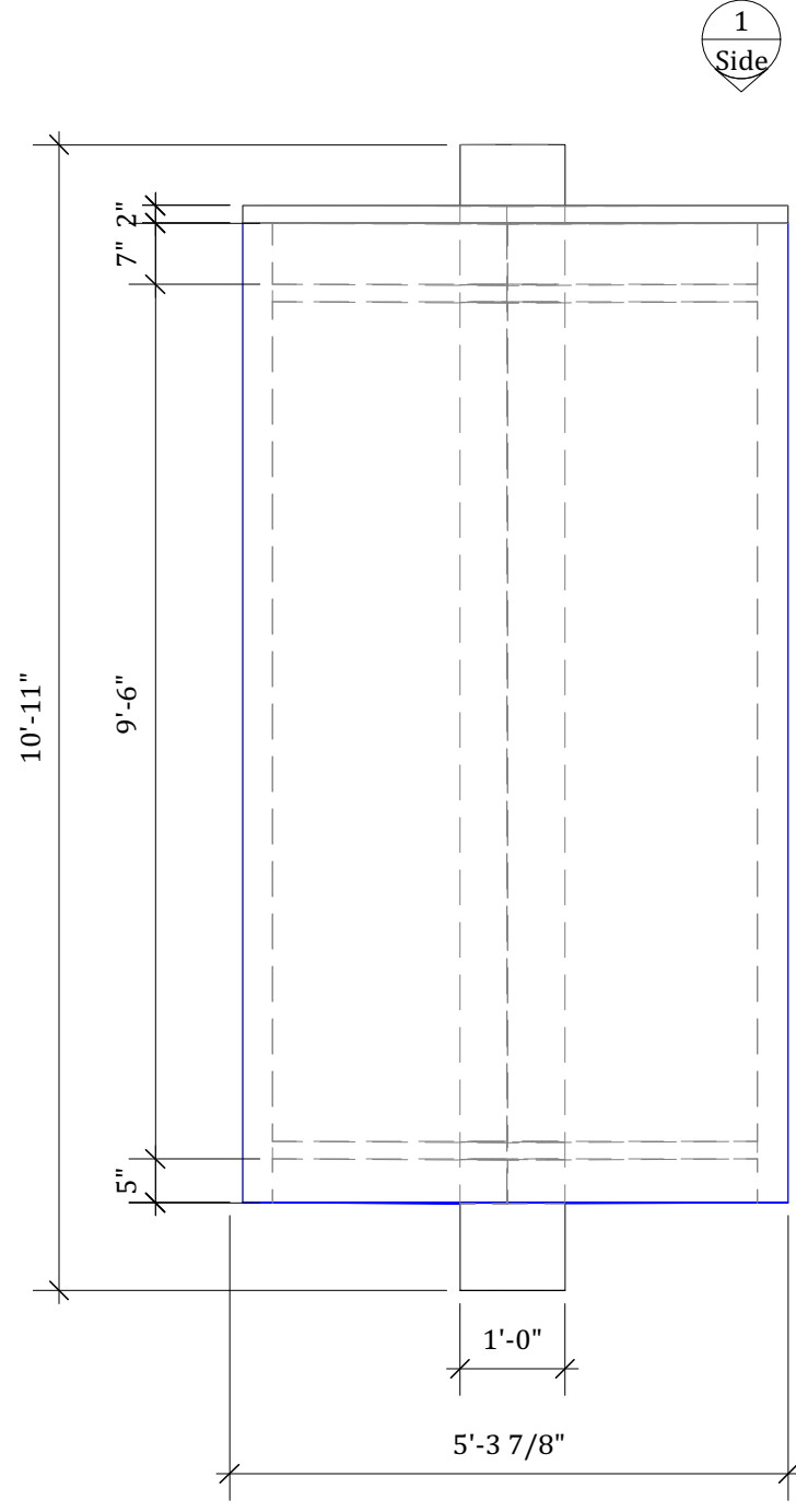
4 S1 Scale: 1/2" = 1'-0"
