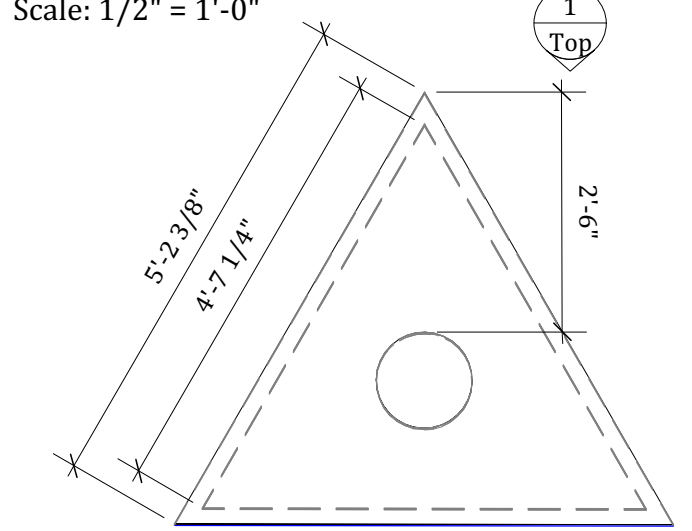
5 S1 Top/Bottom Scale: 1/2" = 1'-0"
